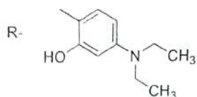
Rhodamine B hydrazide
